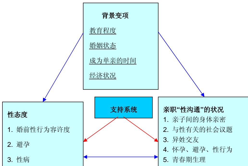
图 1 研究架构图
