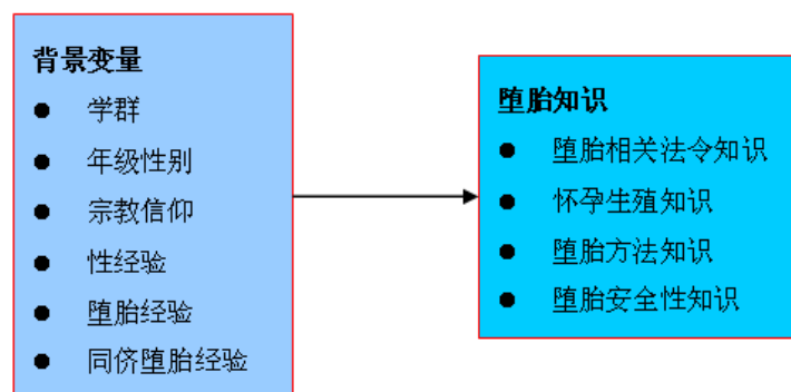
图 1 研究架构
