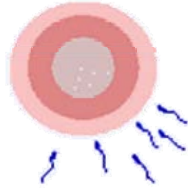
图 4 受精(fertilization)
