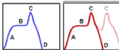
图 2 性反应
